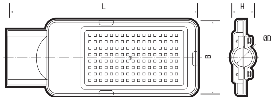
Рис 1. Светильник PSL 08
